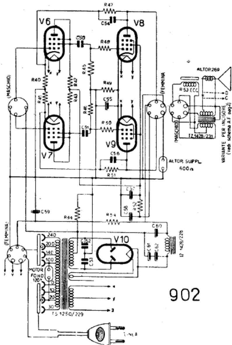
PHONOLA RADIO - Mod. 902 - Amplificatore finale in contropase e alimentatore anodico. Valvole e tensioni:
